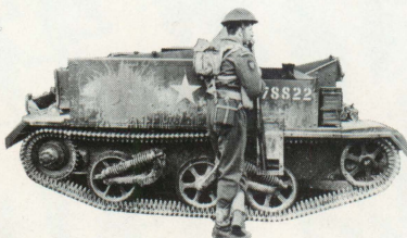
ガーデン・ロイド式ブレンガン・キャリアー (英)機関銃車
